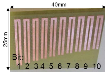
Fig. 3 Chipless RFID Tag
