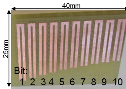
Fig. 3 Chipless RFID Tag
