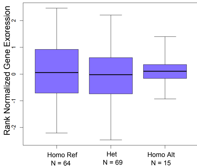
MANBA : rs2720460 2
