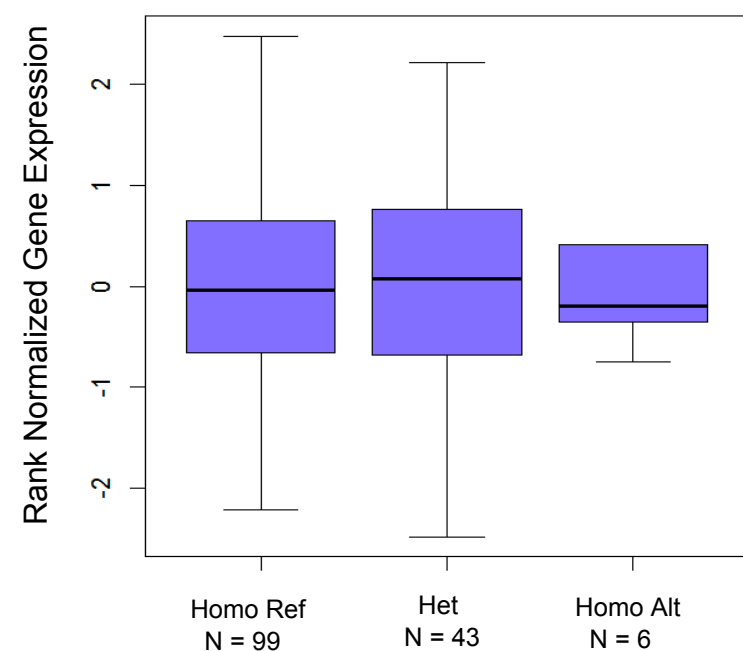
WDR73 : rs2304416 2
