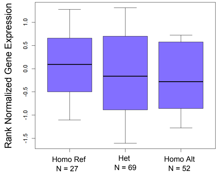
BAK1 : rs210138 2
