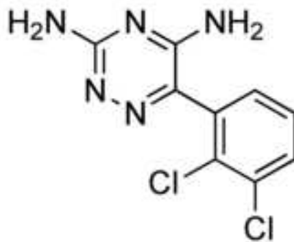
Lamotrigine
